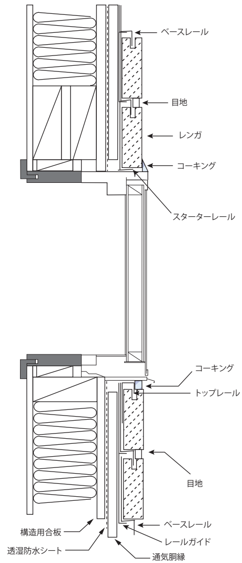
縦断面図
