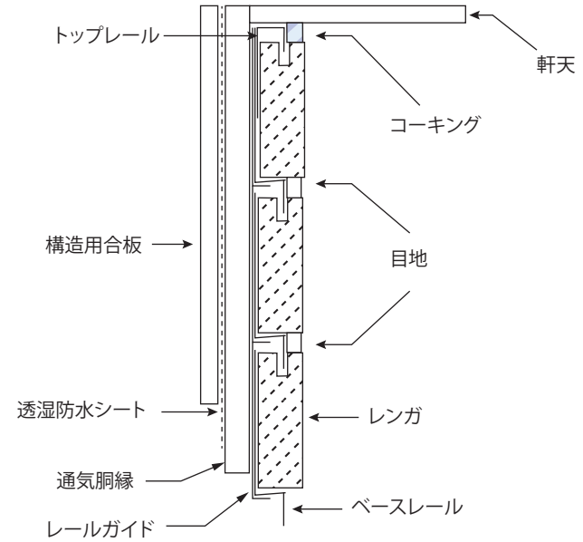
軒天納まり
