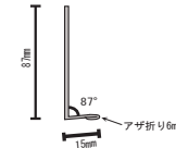
スターターレール (L=2035mm, T=0.35mm)
